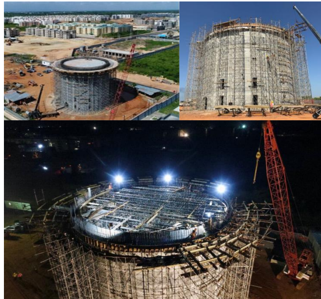
Trabajos en el pedestal de H.A. que soportará el tanque de agua del proyecto Ciudad Juan Bosch
