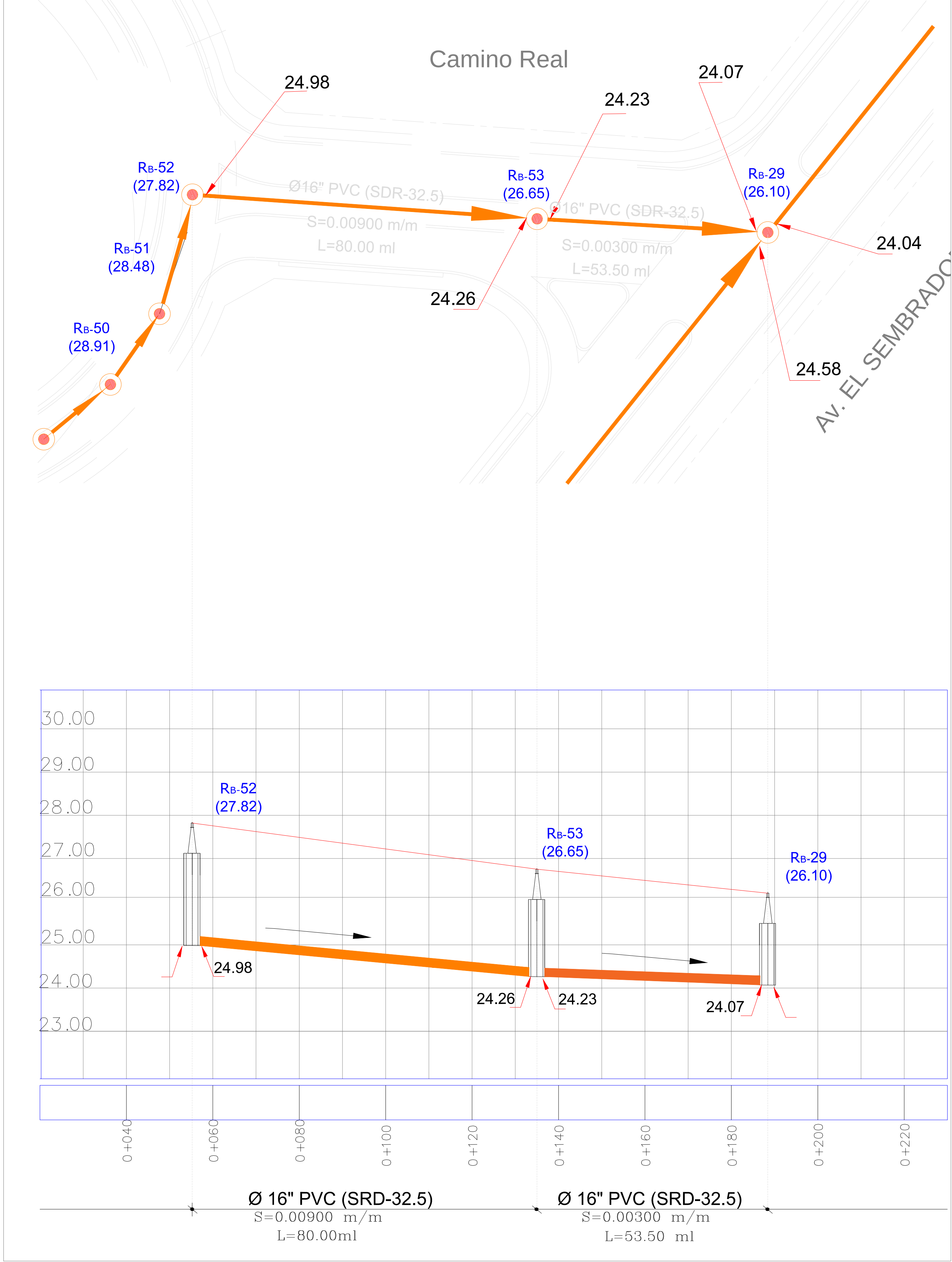
PERFIL LONGITUDINAL AV. CAMINO REAL, Desde RB-52 Hasta RB-29
