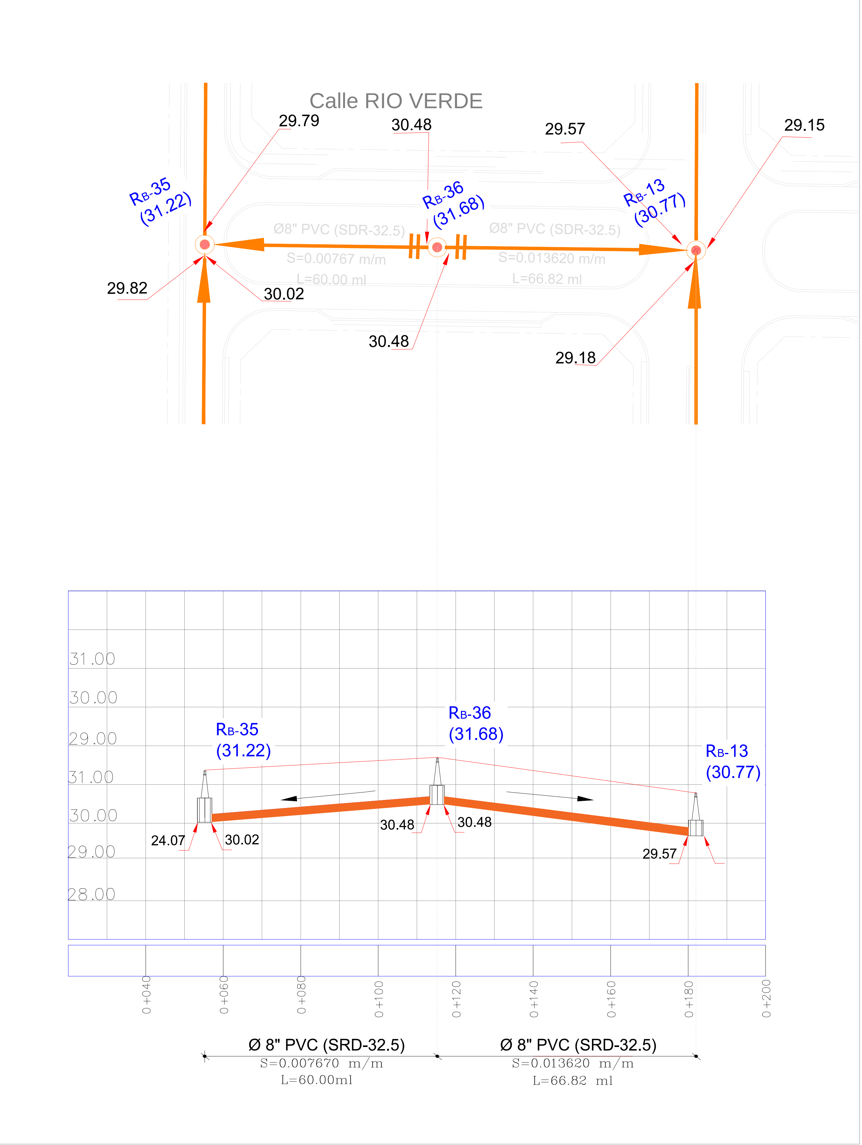
PERFIL LONGITUDINAL CALLE RIO VERDE, Desde RB-35 hasta RB-13
